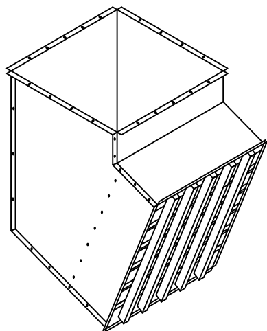
45° DIFFUSER
